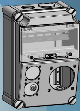
Vario Boxes
